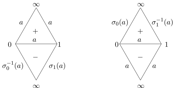
Paramétrisation positive
